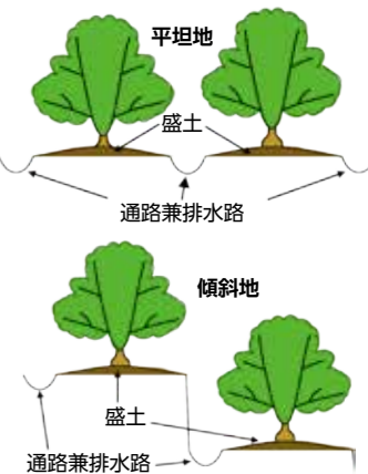
図1. 排水対策
